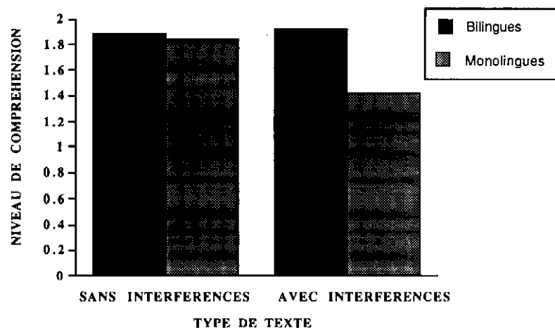
Figure 2 : Niveau moyen de compréhension des sujets bilingues et monolingues lors de la deuxième présentation des deux types de textes - sans interférences et avec interférences
